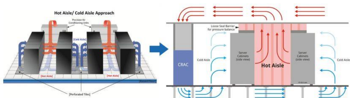
Figuur 27: koude en warme gangen in datacenters
